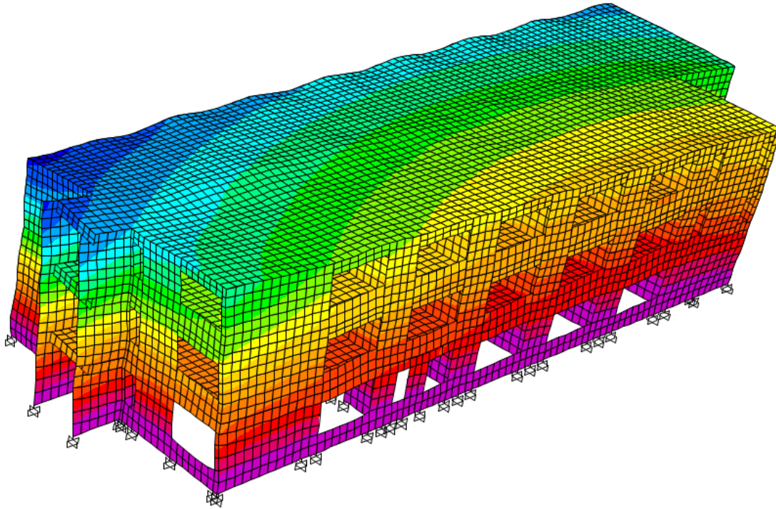
Foto 03 – Moduri proprii de vibrații: Mod 1 ( T=0,16s )- C1
