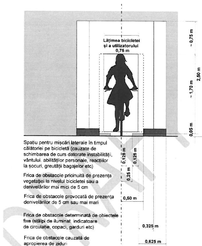
Figura 4. Distanța față de obstacolele din vecinătate
